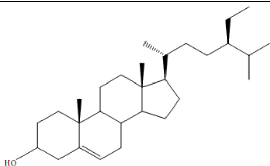
Fig 1. BAL-01 (β- Sitosterol)
